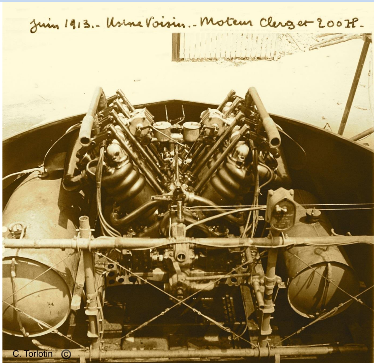
Juin 1913 – Usine Voisin – Moteur Clerget 200 ch
