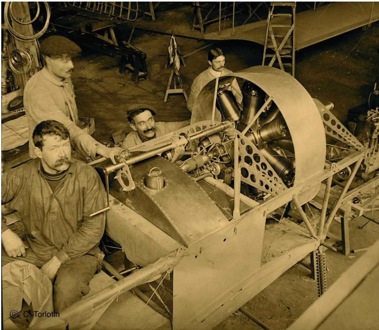
Moteur Gnôme 100 ch – avril 1913
