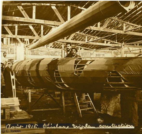
Usine Voisin – août 1916 – construction du fuselage d'un triplan
