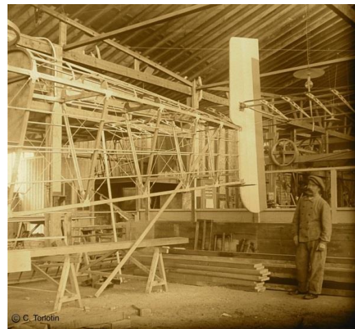
Montage d'un capot et de la partie arrière d'un fuselage
