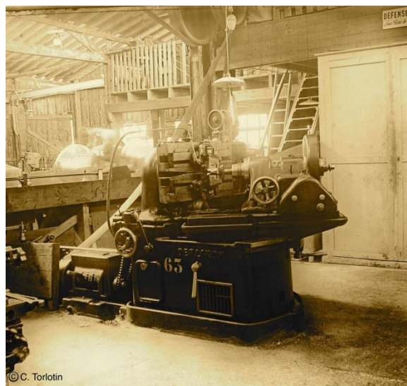
Usine Voisin avril 1913 - Fraiseuses
