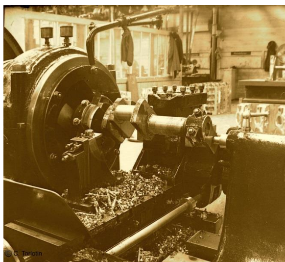
Usine Voisin – Usinage de vilbrequin
